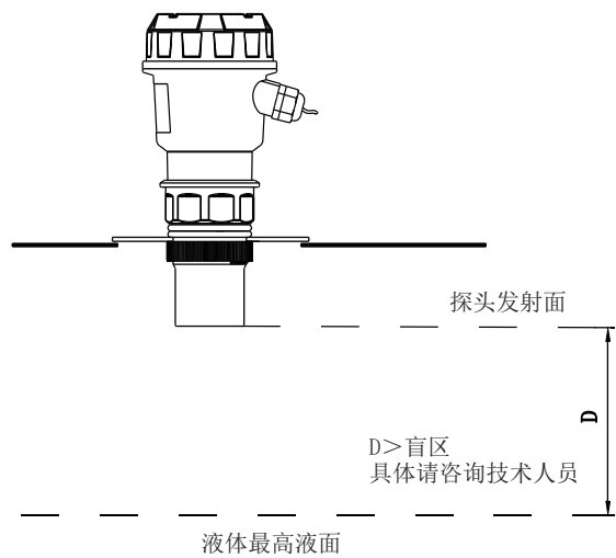
图四 法兰型安装在无接管平顶罐上
