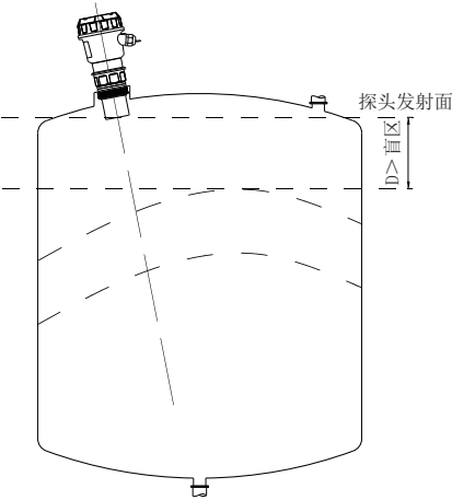
图十二 安装在螺纹接管
